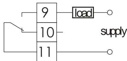
Fig. 6. Control/Alarm output
